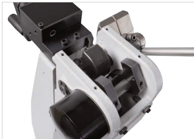
Patentovaná mechanika se strmým nárůstem síly na konci zdvihu
